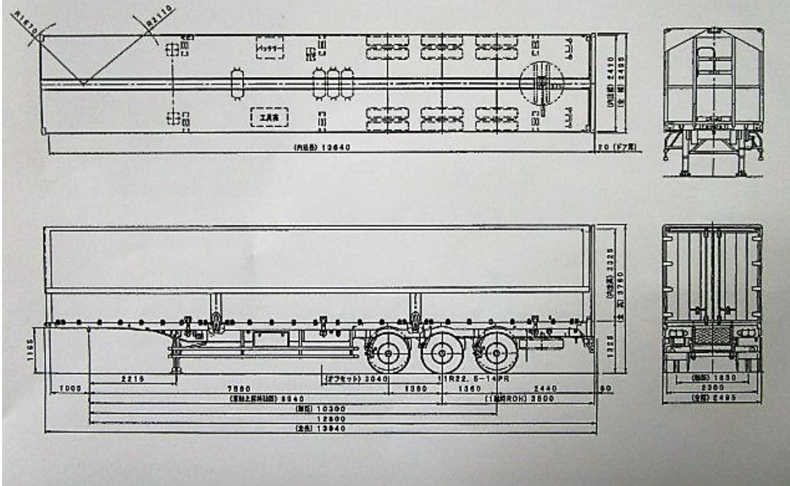
フルハーフ DFPTF341A改型セミトレーラー 外観図
