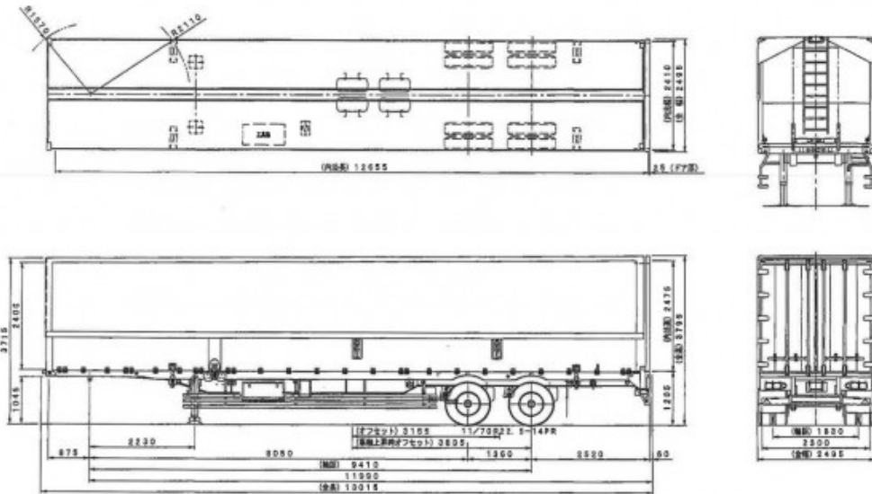
フルハーフ DFPTF241AN改型セミトレーラ 外観図
