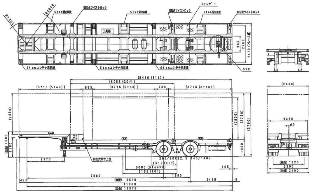
フルハーフ DFPDG241B型セミトレーラ 外観図
