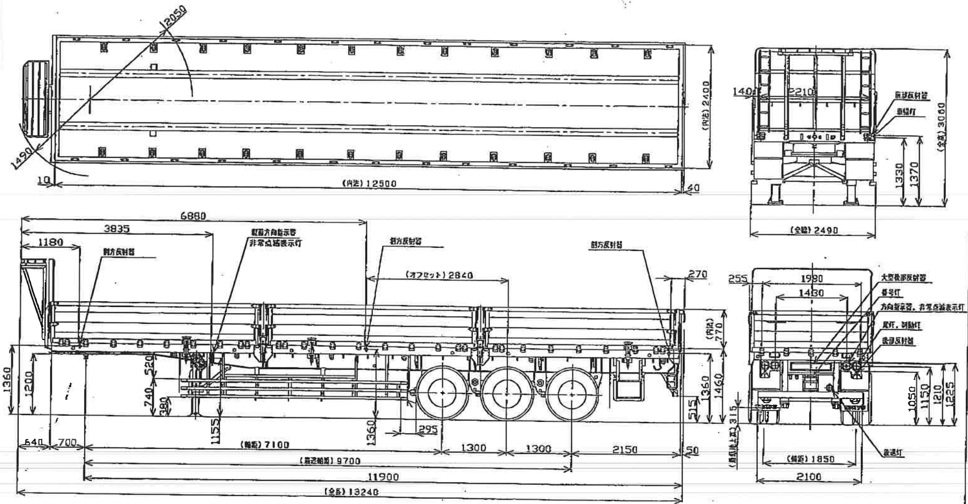
東急TF36H4C3S型セミトレーラ外観四面図
