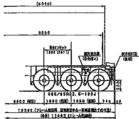
部分図3：フレーム収縮時の側面図 (後部のみ)
