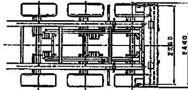
部分図2：フレーム収縮時の平面図 (後部のみ)
