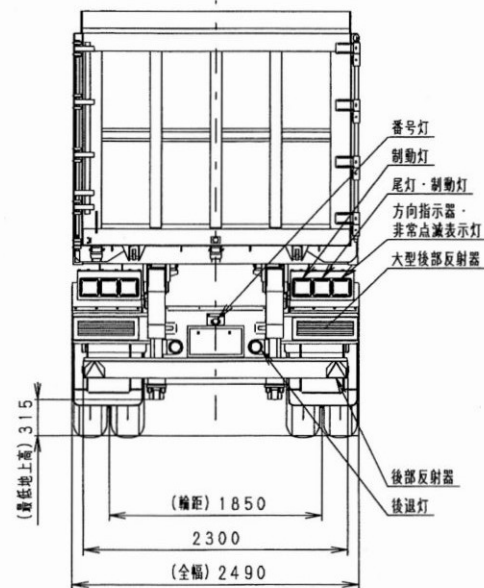
東邦TF36H2C3改型 ダンプセミトレーラ外観四面図
