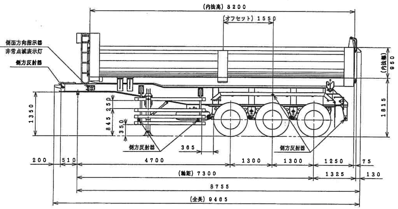
コダイラ KFL32改 ダンプセミトレーラ外観四面図
